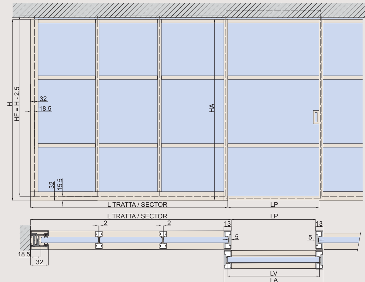
Anta intelaiata "Divina"
