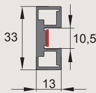
DIV-202 Profilo di finitura
