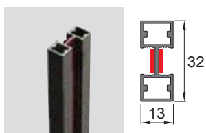
DIV-208 Profilo "H" vetro-vetro
