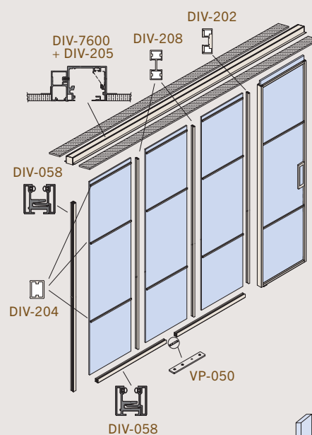
Anta intelaiata "Divina"
