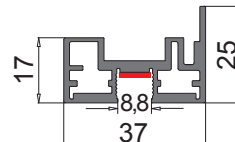
④ DIV-104 MONTANTE VERTICALE (porta doppia lato contropiastra)
