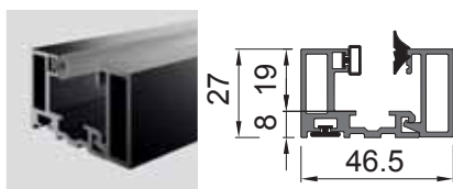
DIV-050 Profilo a scatto per vetro fisso
