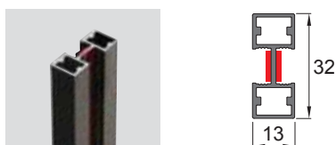
DIV-208 Profilo "H" vetro-vetro
