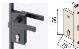
⑩ V-741 PZ SERRATURA VERTICALE
