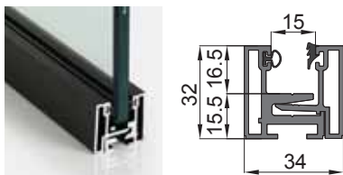
DIV-058 Profilo a scatto per vetro fisso
