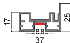
④ DIV-104 MONTANTE VERTICALE (porta doppia lato contropiastra)
